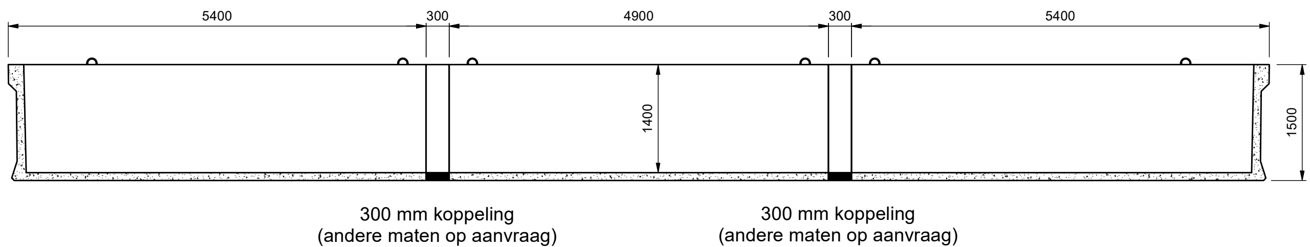
Langsdoorsnede
