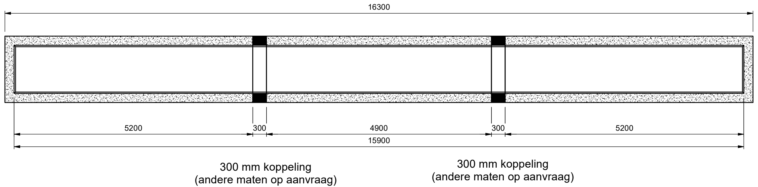
Bovenaanzicht
