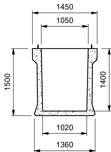
Dwarsdoorsnede
