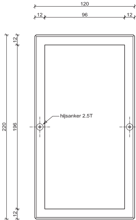
bovenaanzicht put
