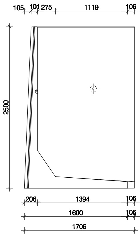
Zijaanzicht
