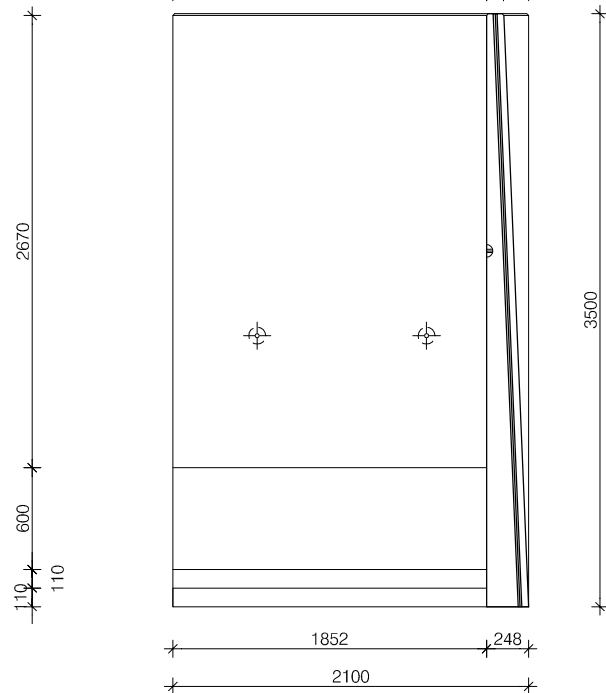
Vooraanzicht
