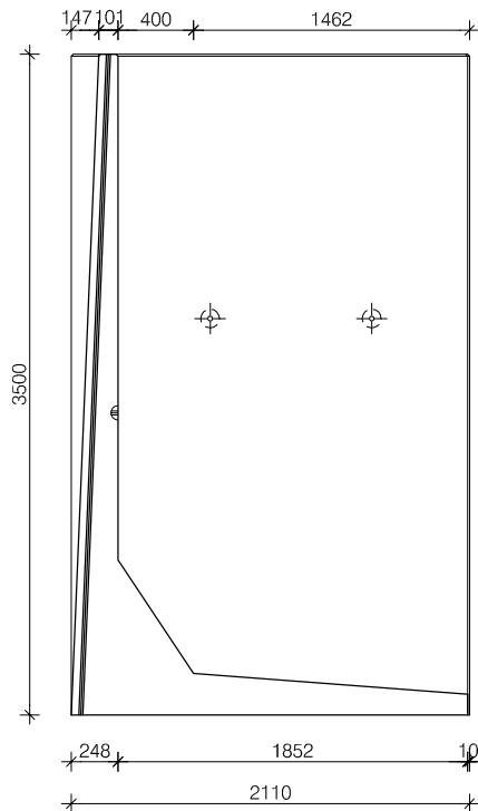
Zijaanzicht
