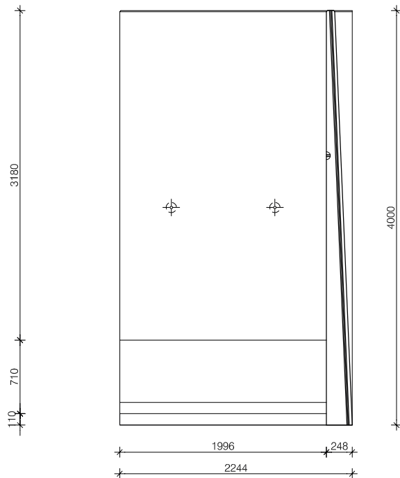
Vooraanzicht
