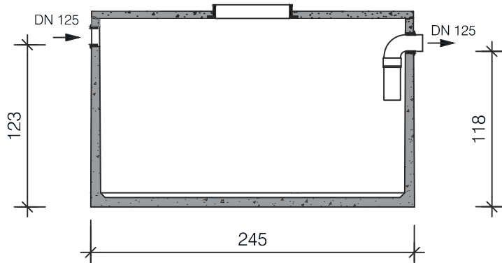
Langsdoorsnede
