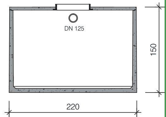
Dwarsdoorsnede
