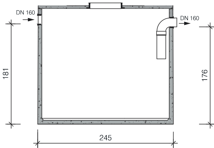
Langsdoorsnede
