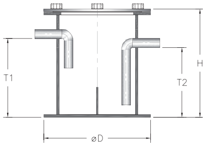
Dwarsdoorsnede
