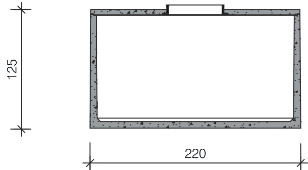
Dwarsdoorsnede
