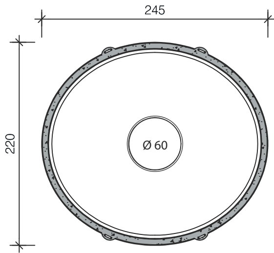
Doorsnede
