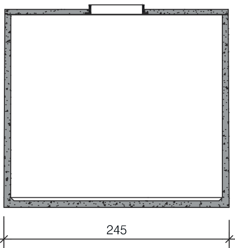
Langsdoorsnede
