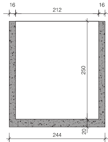
Dwarsdoorsnede
