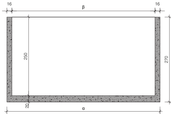
Langsdoorsnede
