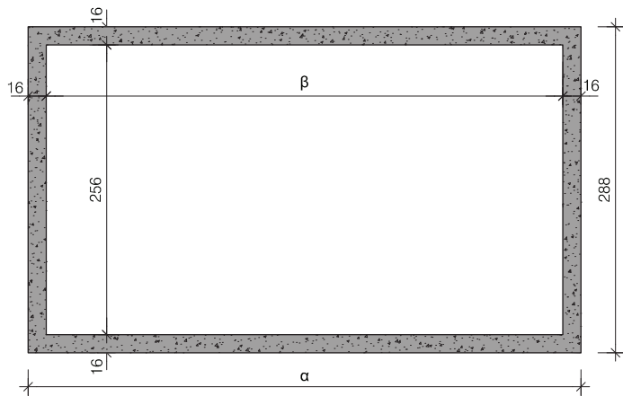
Doorsnede
