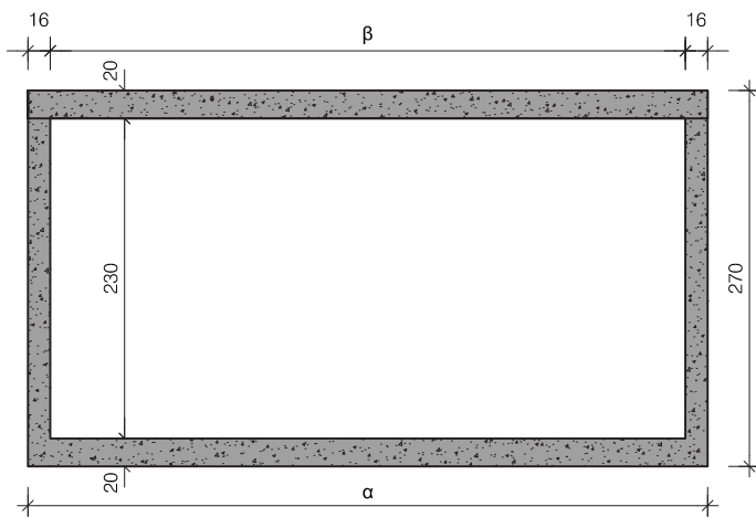
Langdoorsnede
