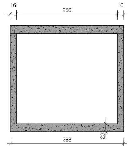
Dwarsdoorsnede
