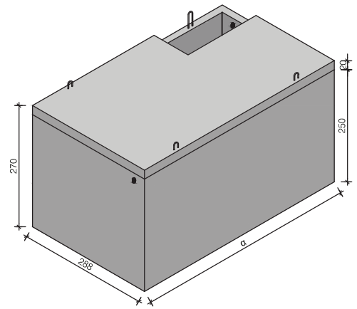
Aanzicht
