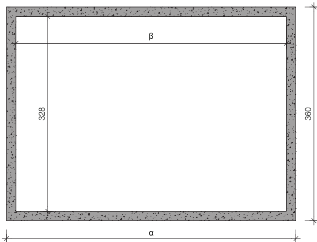
Doorsnede
