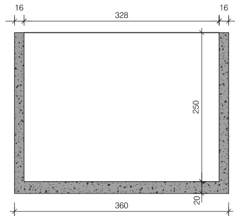
Dwarsdoorsnede
