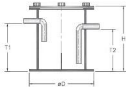
Dwarsdoorsnede
