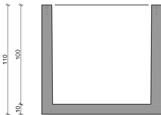
dwarsdoorsnede
