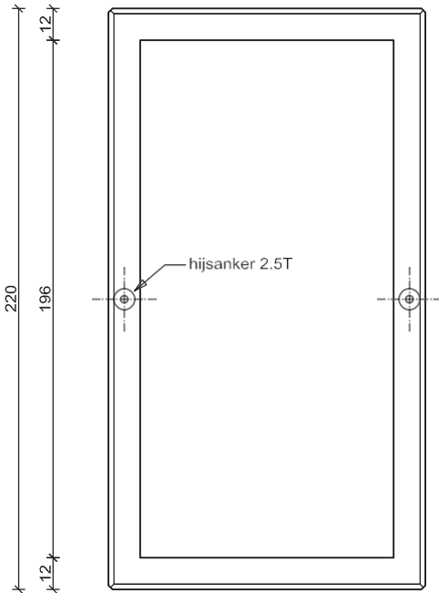
bovenaanzicht put
