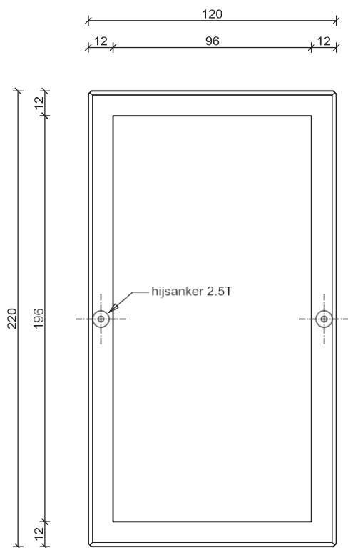
bovenaanzicht put
