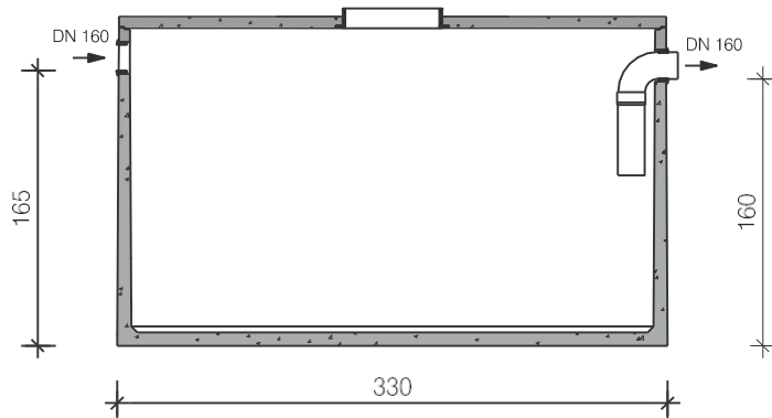
Langsdoorsnede
