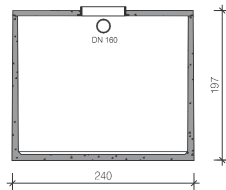
Dwarsdoorsnede
