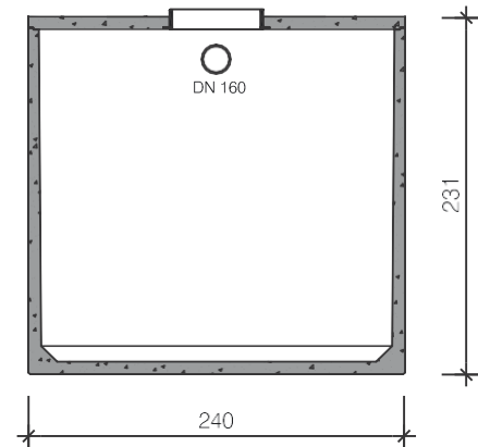
Dwarsdoorsnede
