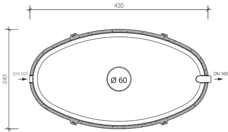
Doorsnede
