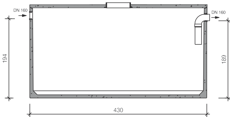
Langsdoorsnede
