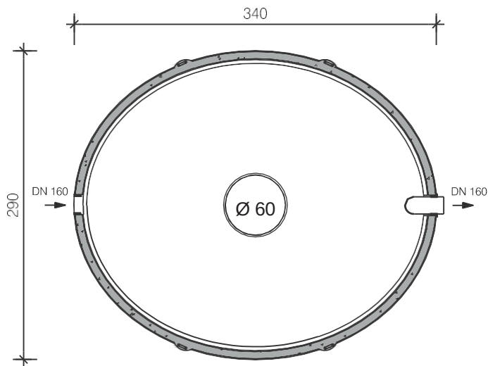
Doorsnede
