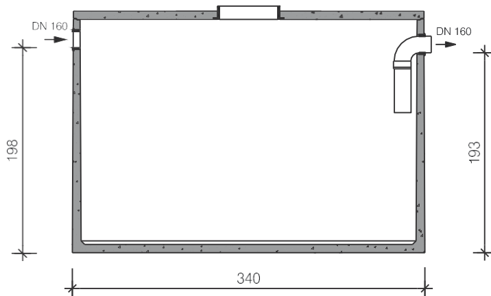
Langsdoorsnede
