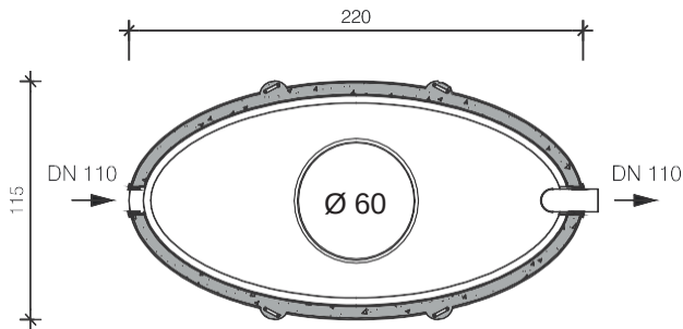
Doorsnede
