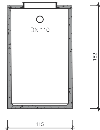
Dwarsdoorsnede
