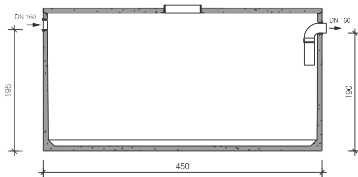
Langsdoorsnede
