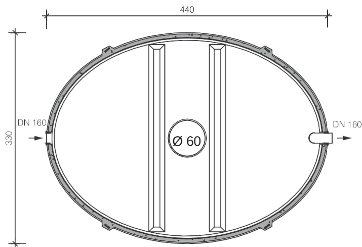
Doorsnede
