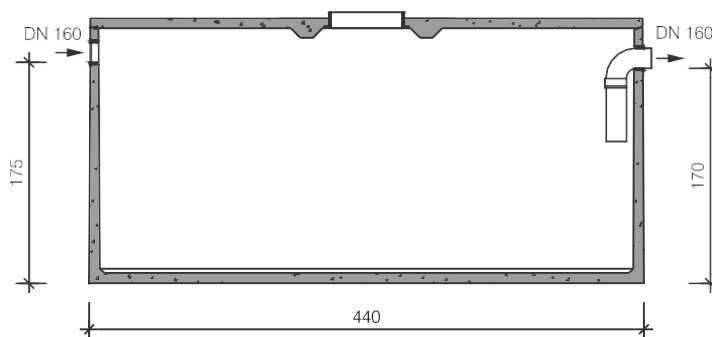
Langdoorsnede
