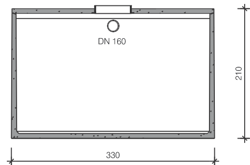
Dwarsdoorsnede
