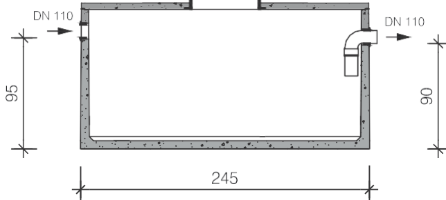
Langsdoorsnede
