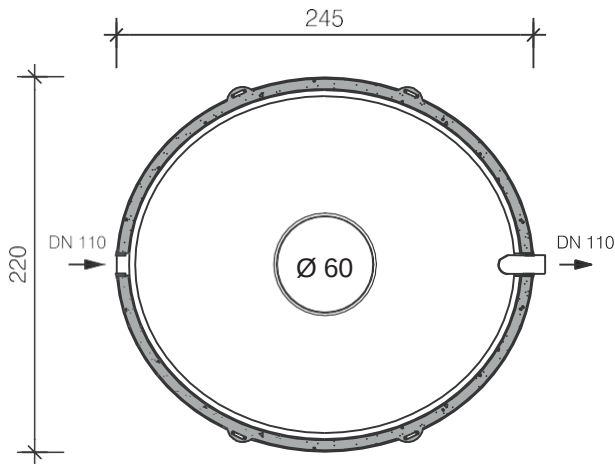
Doorsnede
