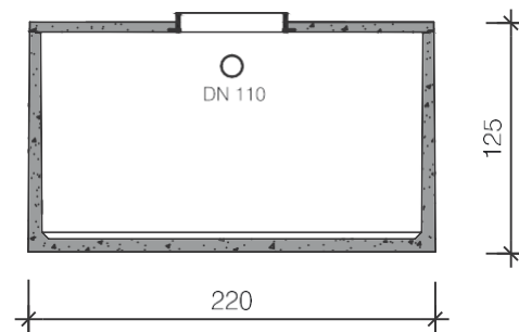
Dwarsdoorsnede
