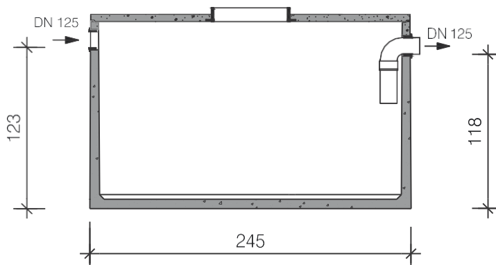
Langsdoorsnede
