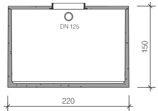
Dwarsdoorsnede
