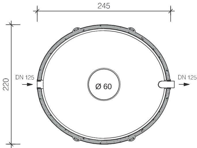
Doorsnede
