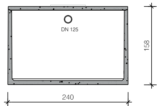
Dwarsdoorsnede
