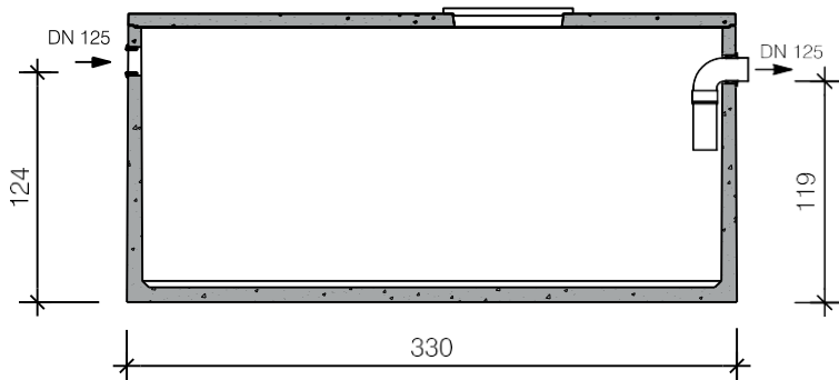
Langsdoorsnede
