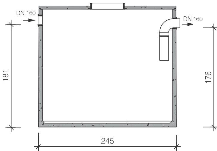
Langsdoorsnede
