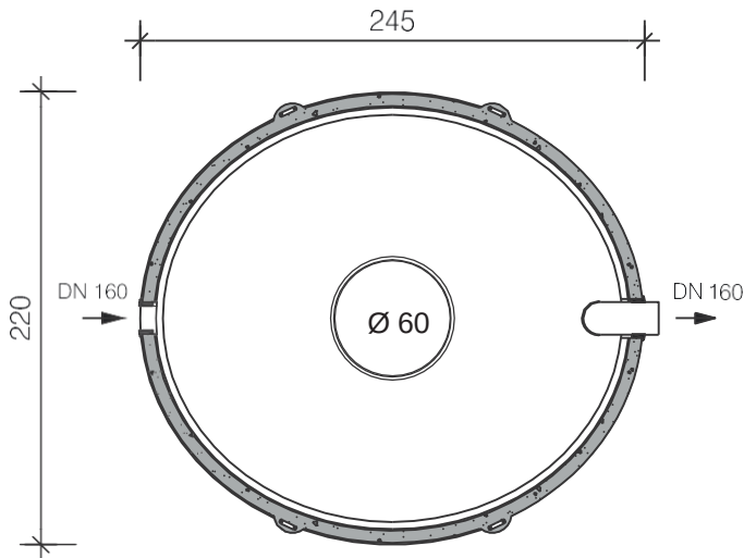
Doorsnede
