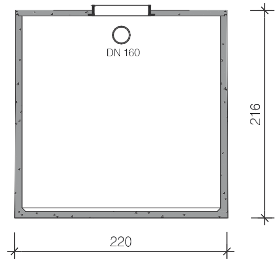
Dwarsdoorsnede
