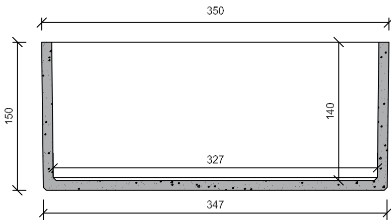
Langsdoorsnede
