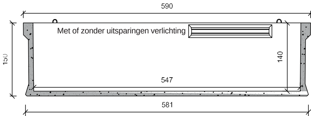
Langsdoorsnede
