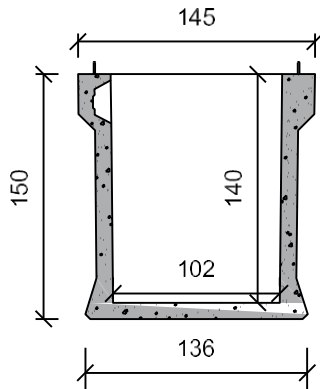
Dwarsdoorsnede
