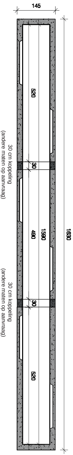
Bovenaanzicht
