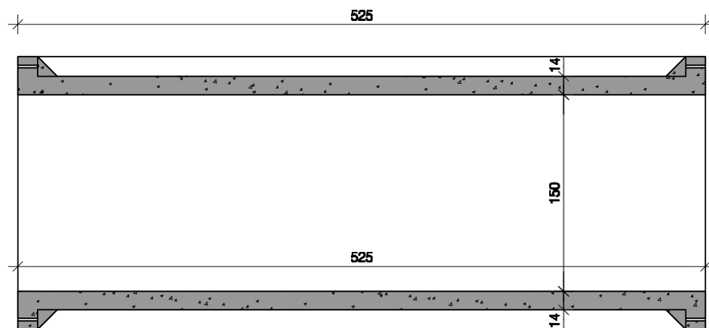
Langdoorsnede
