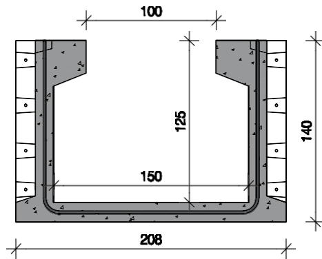
Doorsnede
