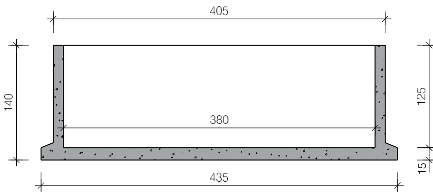
Langsdoorsnede
