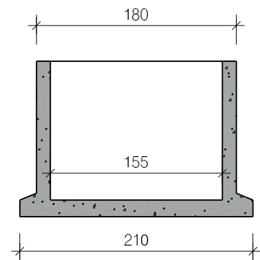
Dwarsdoorsnede
