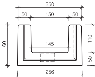
vooraanzicht goot
