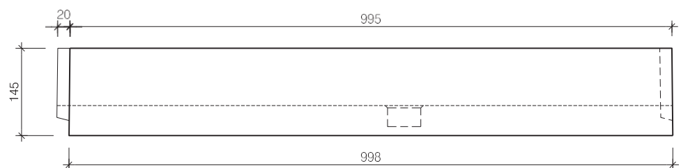
zijaanzicht goot
