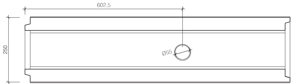
bovenaanzicht goot
