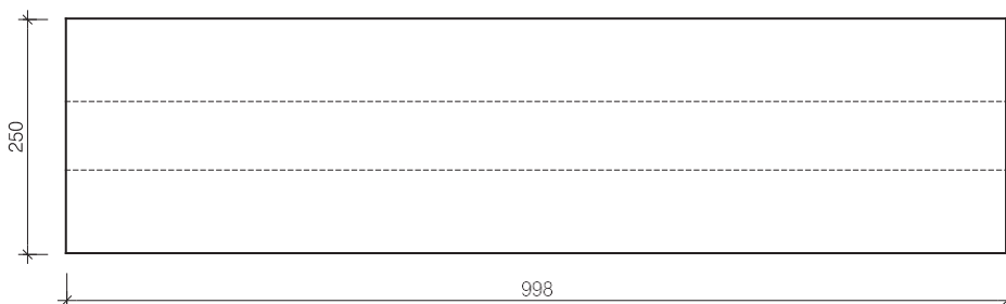
bovenaanzicht deksel
