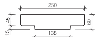
vooraanzicht deksel
