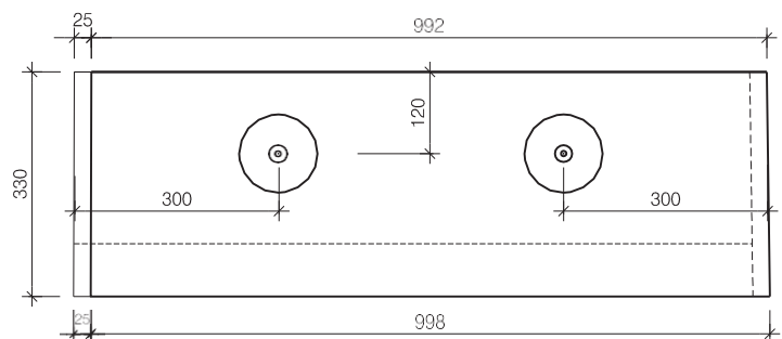
zijaanzicht goot
