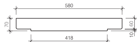
vooraanzicht deksel
