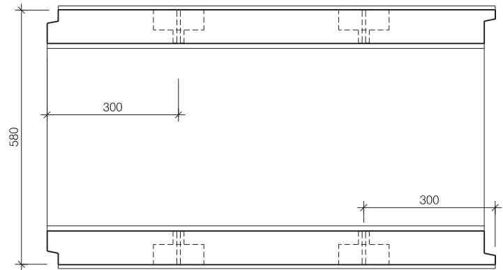
bovenaanzicht goot
