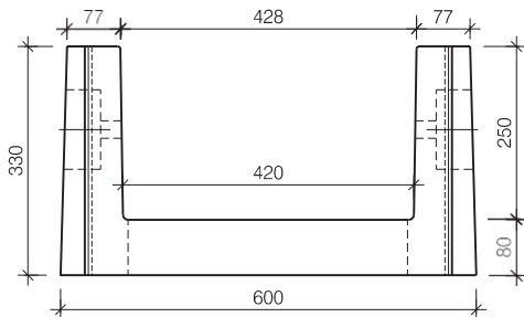
vooraanzicht goot
