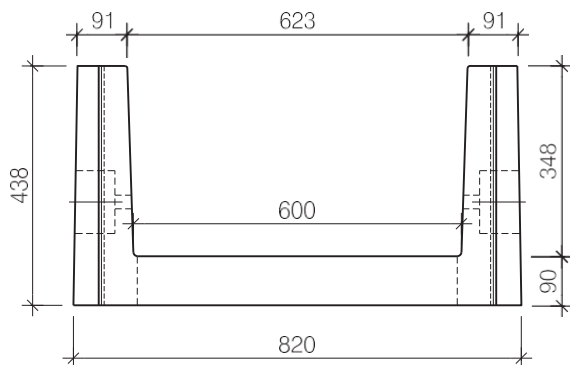
vooraanzicht goot
