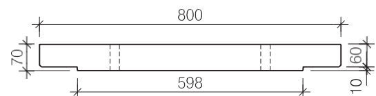
vooraanzicht deksel
