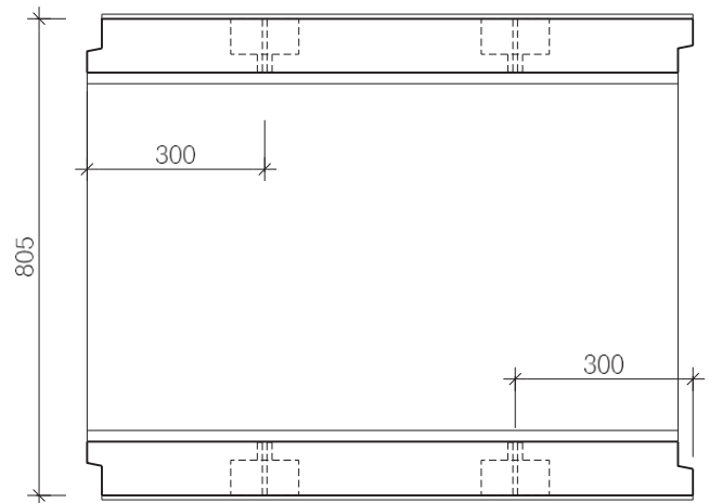
bovenaanzicht goot
