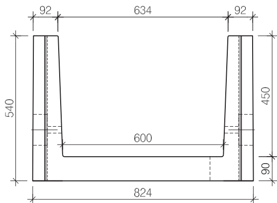
vooraanzicht goot
