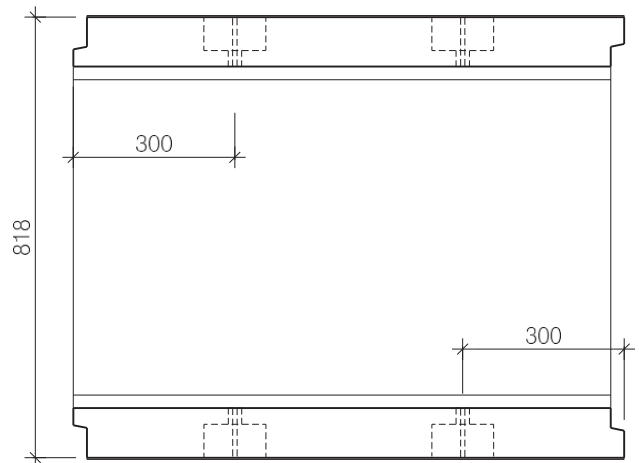
bovenaanzicht goot
