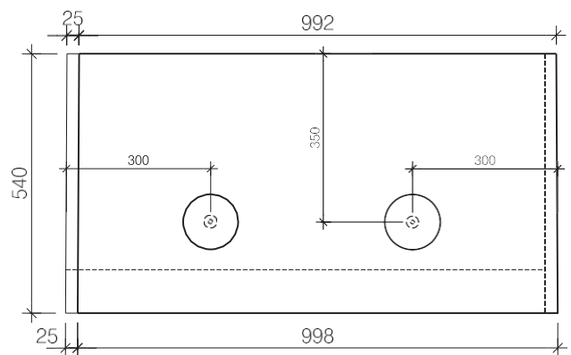
zijaanzicht goot
