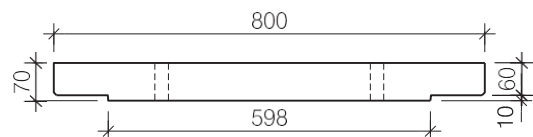
vooraanzicht deksel
