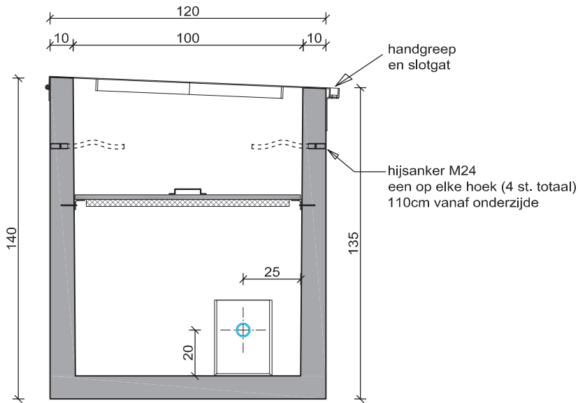
dwarsdoorsnede
